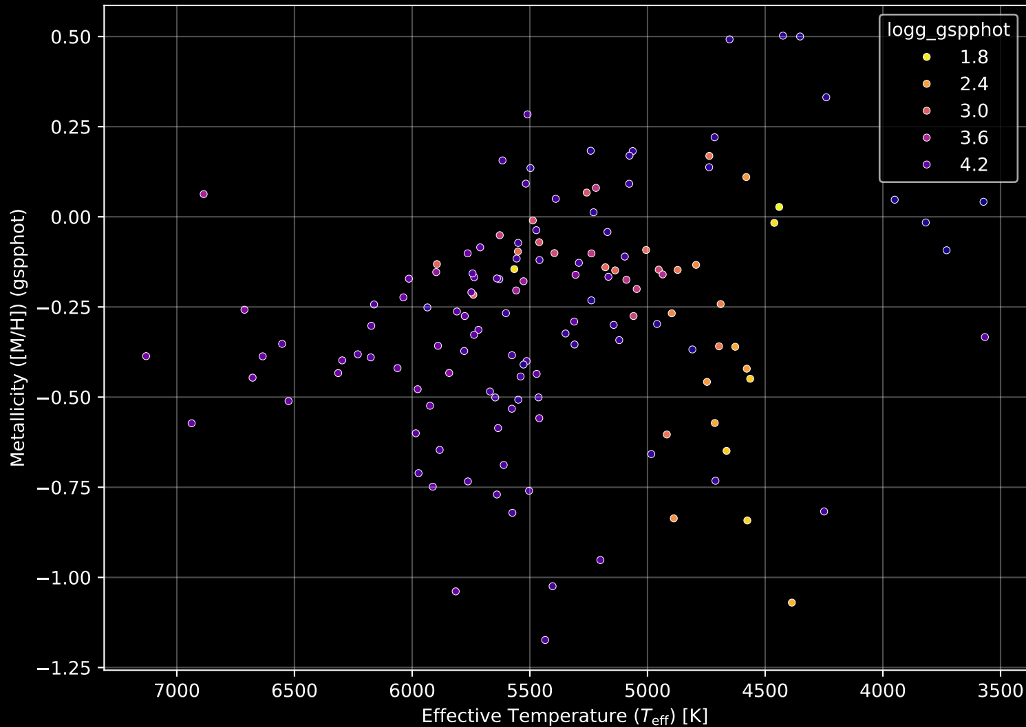
APOGEE DR17 Field: [042+43_MGA] Stellar Population Parameters (n= 142)
